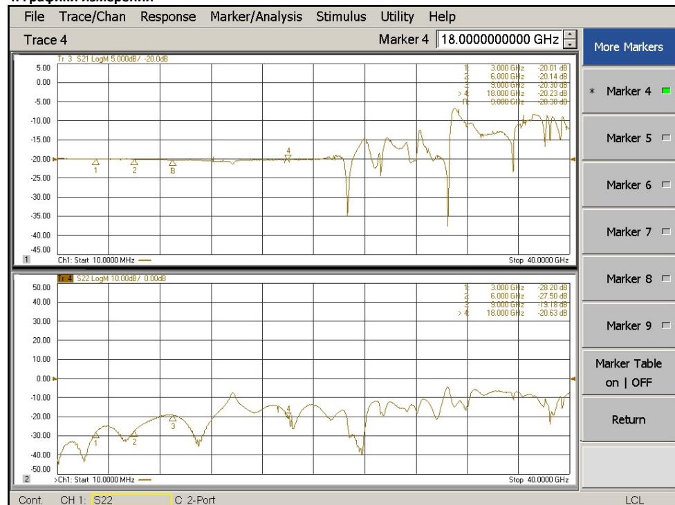
Графики для АЧХ при отсчётном уровне равном -20 дБ и 0 дБ
